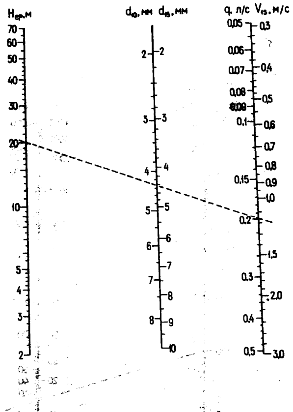
Черт. 6. Номограмма для определения диаметров отверстий диафрагм, устанавливаемых у смесителей водоразборной арматуры санитарных приборов d_{10}(d_{15}) — диаметр отверстия диафрагмы, мм, устанавливаемой в соединительных патрубках (подводках) смесительной водоразборной арматуры с условным проходом d = 10 и 15 мм; v_{15} — скорость движения воды, м/с, в подводке d = 15 мм
